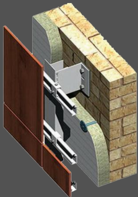
Навесная система крепления (аграфы)
