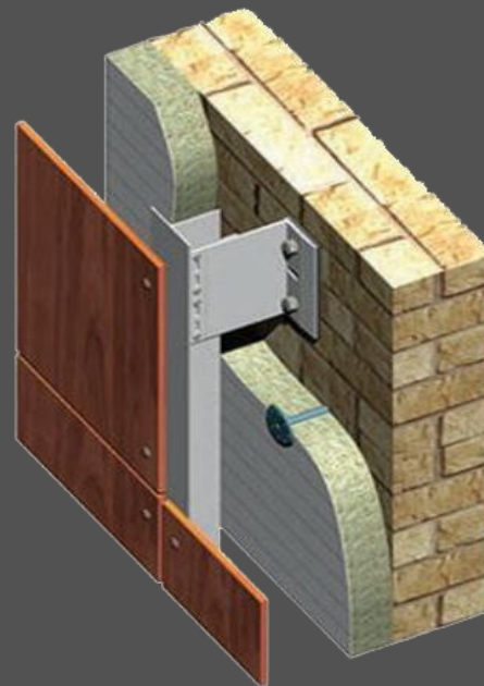
Крепление на заклепки
